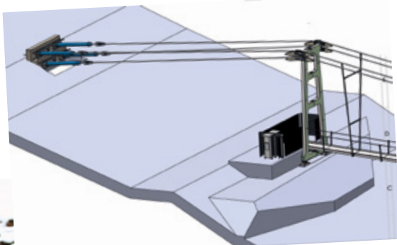
Die Skizze zeigt eine Darstellung des Brückenbauwerks an der Seite der Mühlenkopfschanze.
